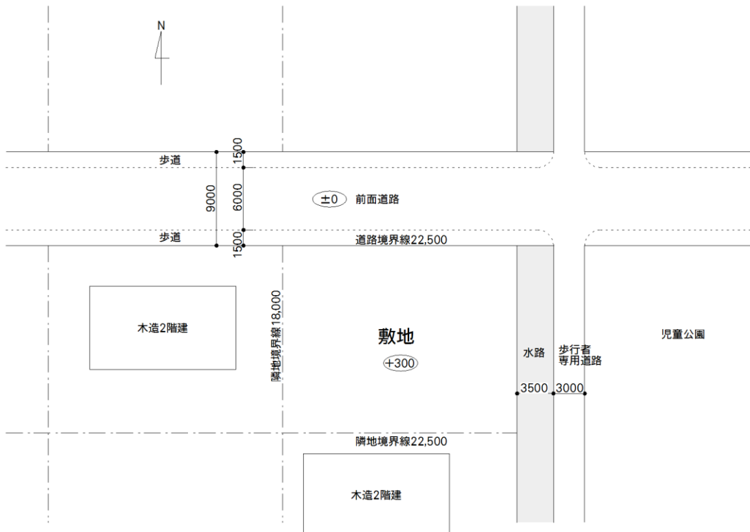
敷地図
